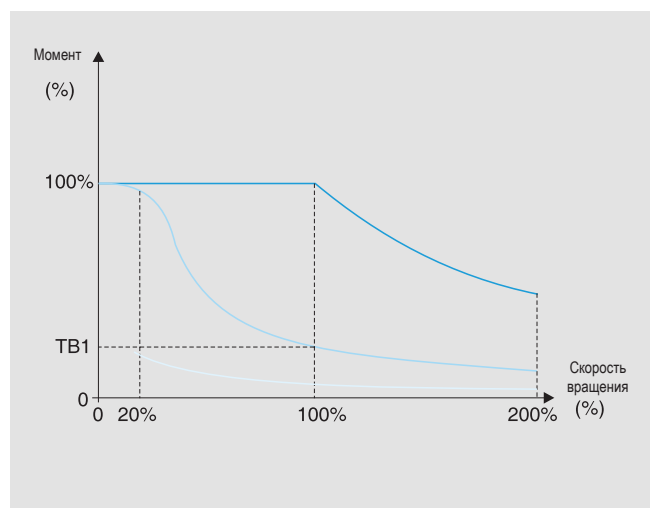
Кривые зависимости моментов от скорости для двигателей приводимых ПЧ CFW-09
