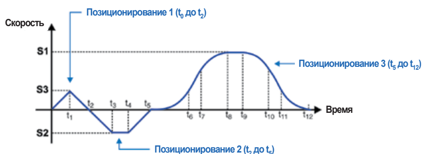
Пример использования PLC1 и PLC2
