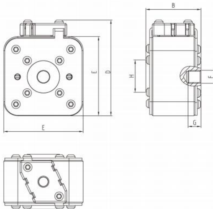
【Fig.-7G3A】 Unit:mm
