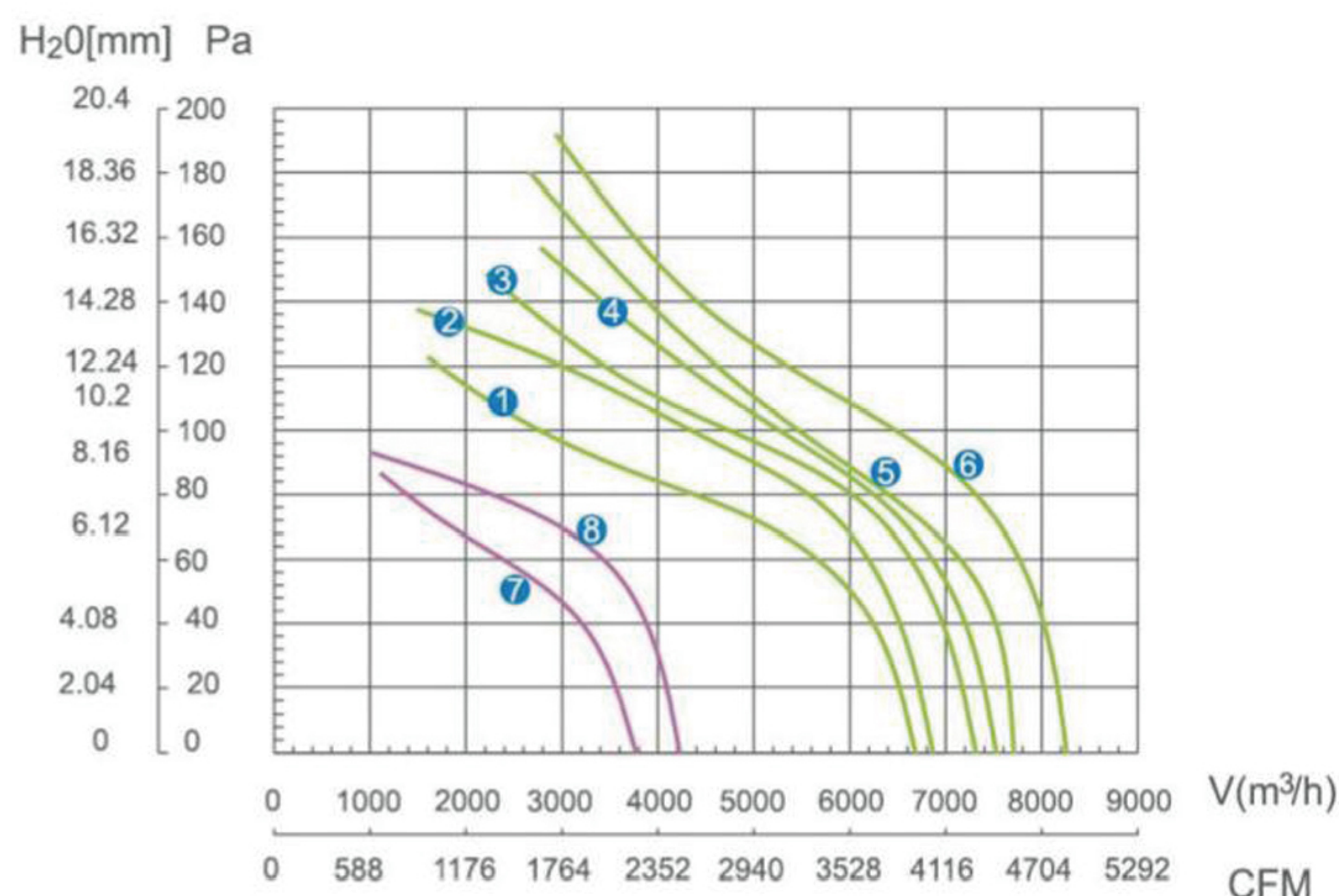
曲线图 Graph
