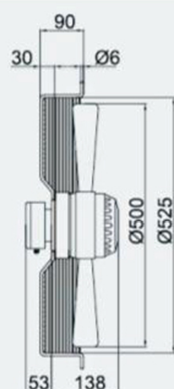
安装尺寸图 Mounting dimensions
