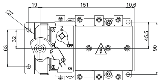
Вид спереди
